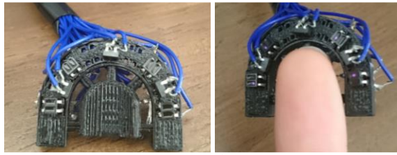
図1 指先装着型デバイスの外観
