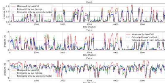
図9 ある被験者における3次元接触力推定結果
